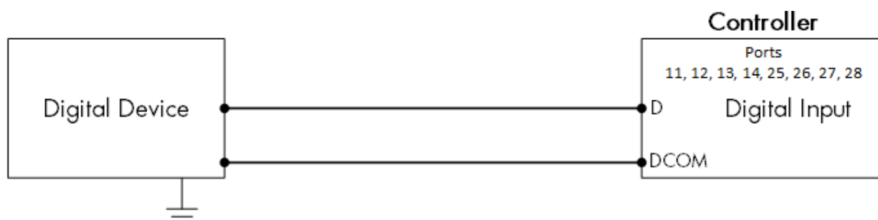
图 20：数字设备接线图（转换文本）
