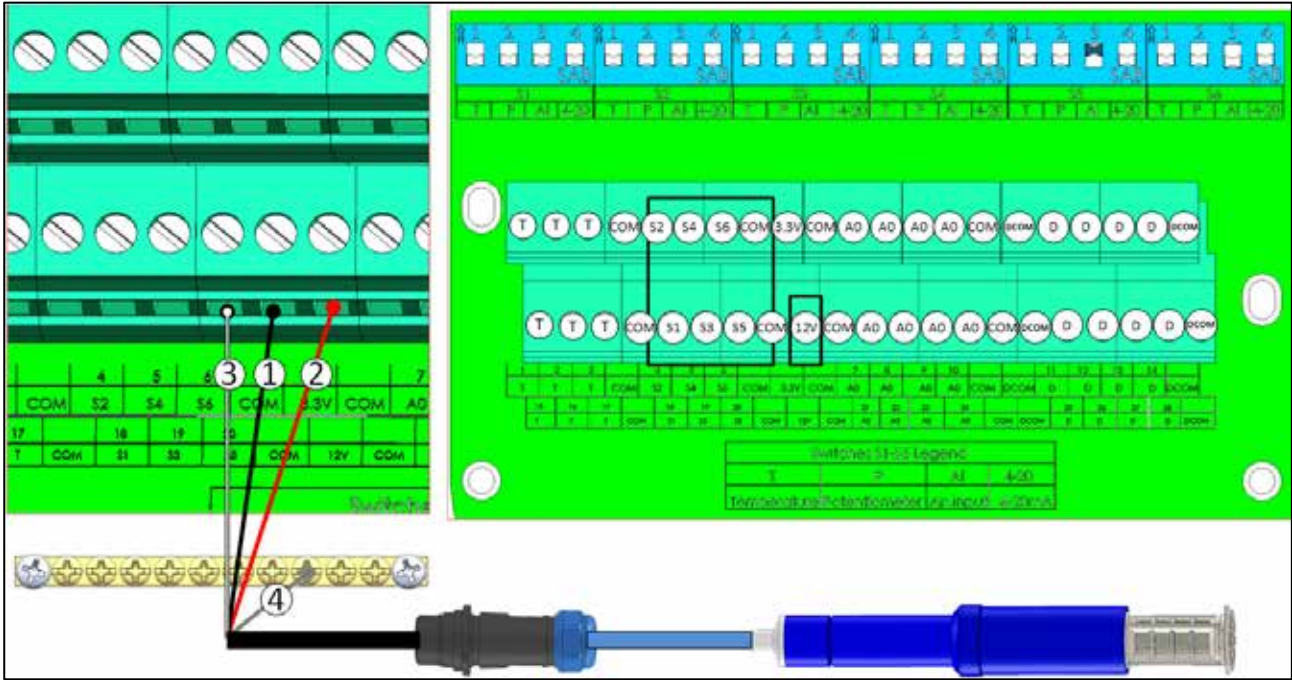
图 27：RHS+布线
