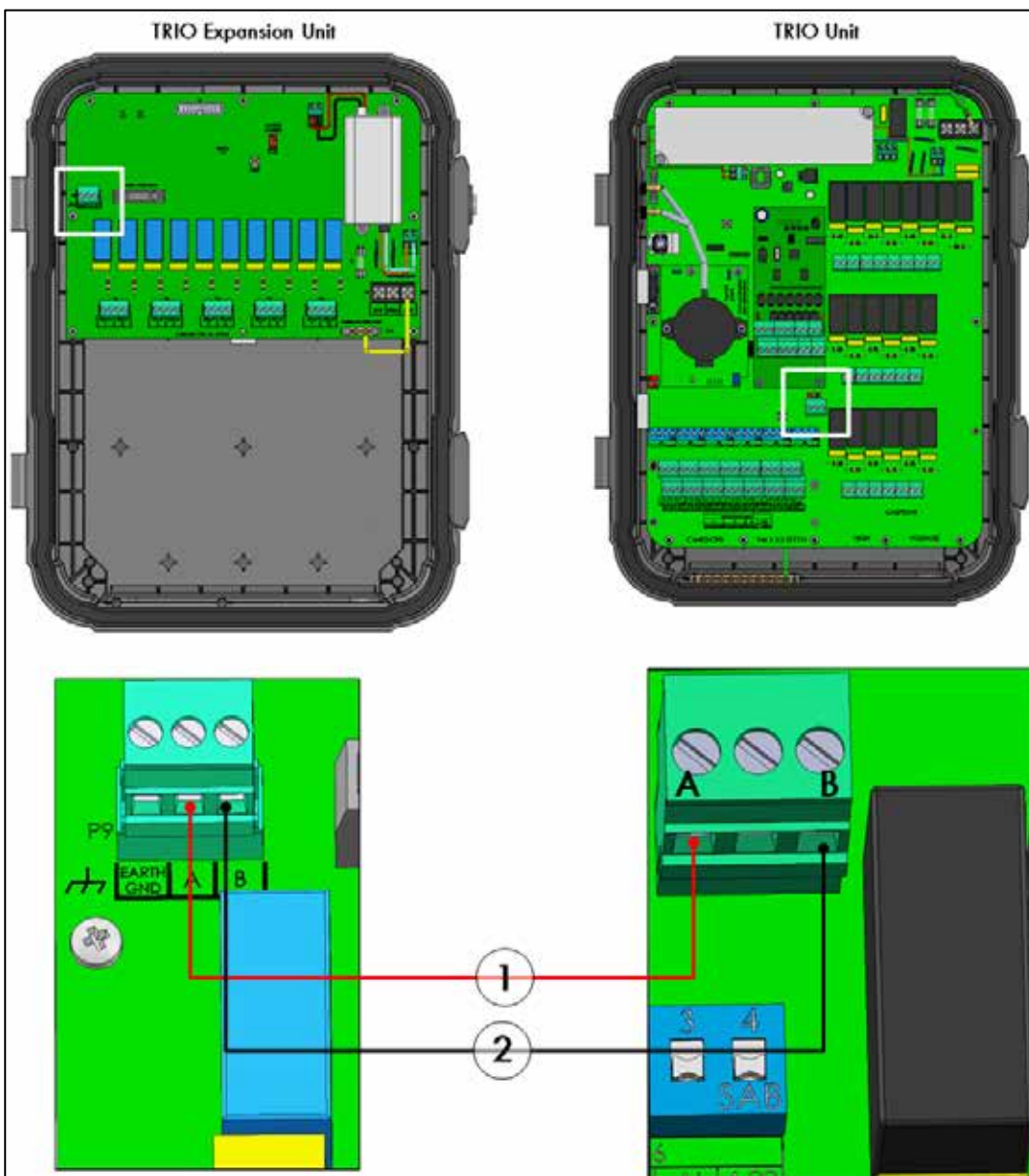
图 48：接线图
