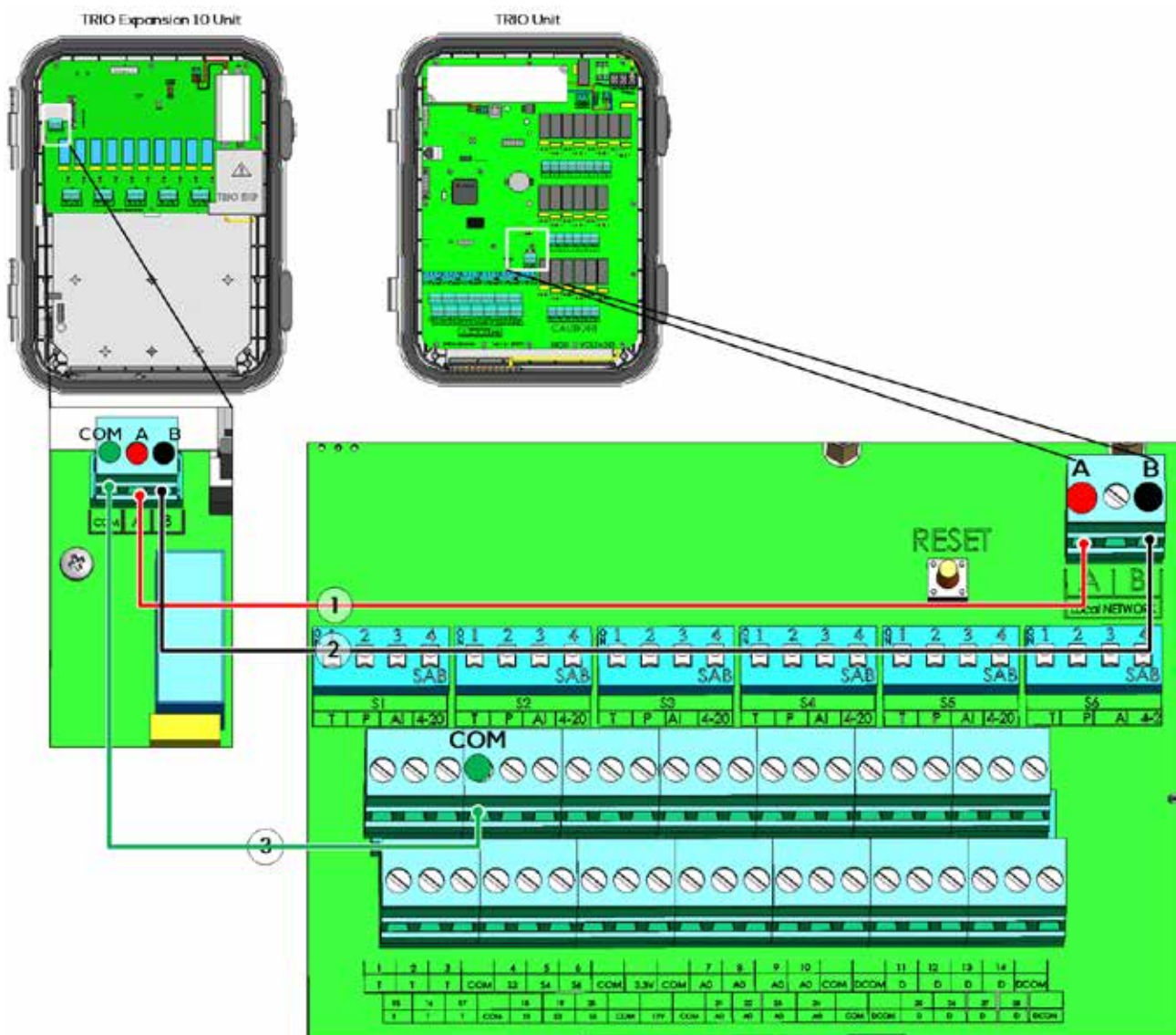
图 65： 面板安装/扩展面板安装接线
