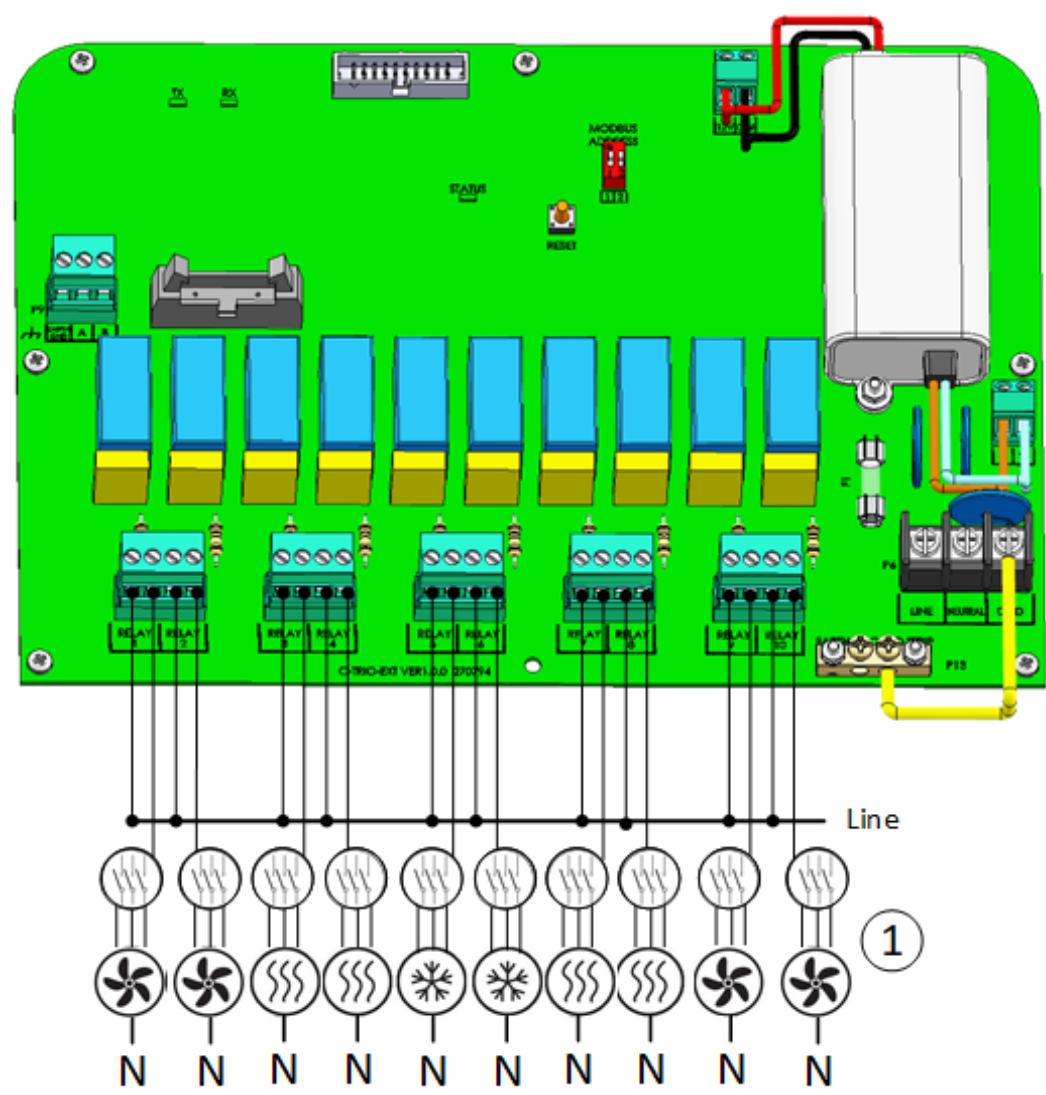
图 50： 高压设备 ( 示例 )
