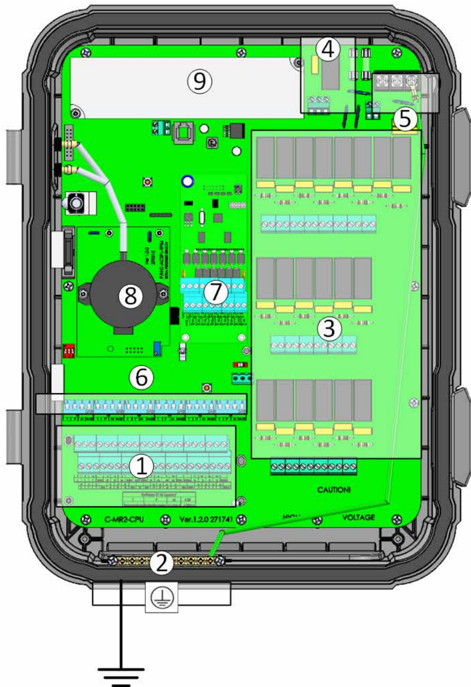
图 6：主要板布局
