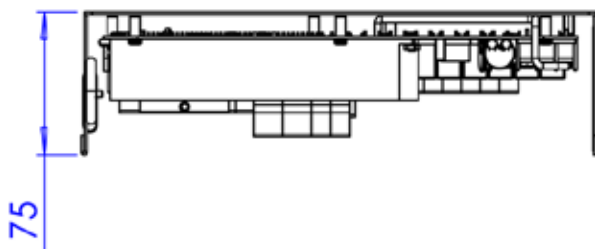
图 64：后面板深度尺寸
