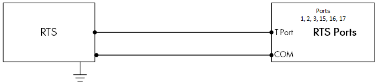
图 24：RTS接线图
