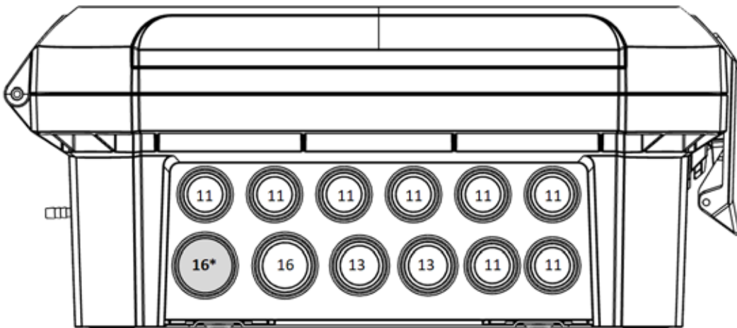
图 3：鸡管家TRI0预留挡片和PG螺纹尺寸
