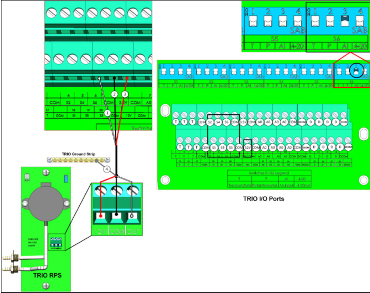
图 36 : RPS接线
