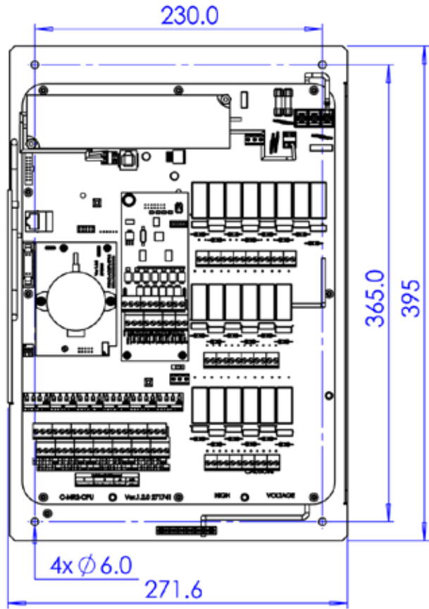
图 56: 后面板尺寸
