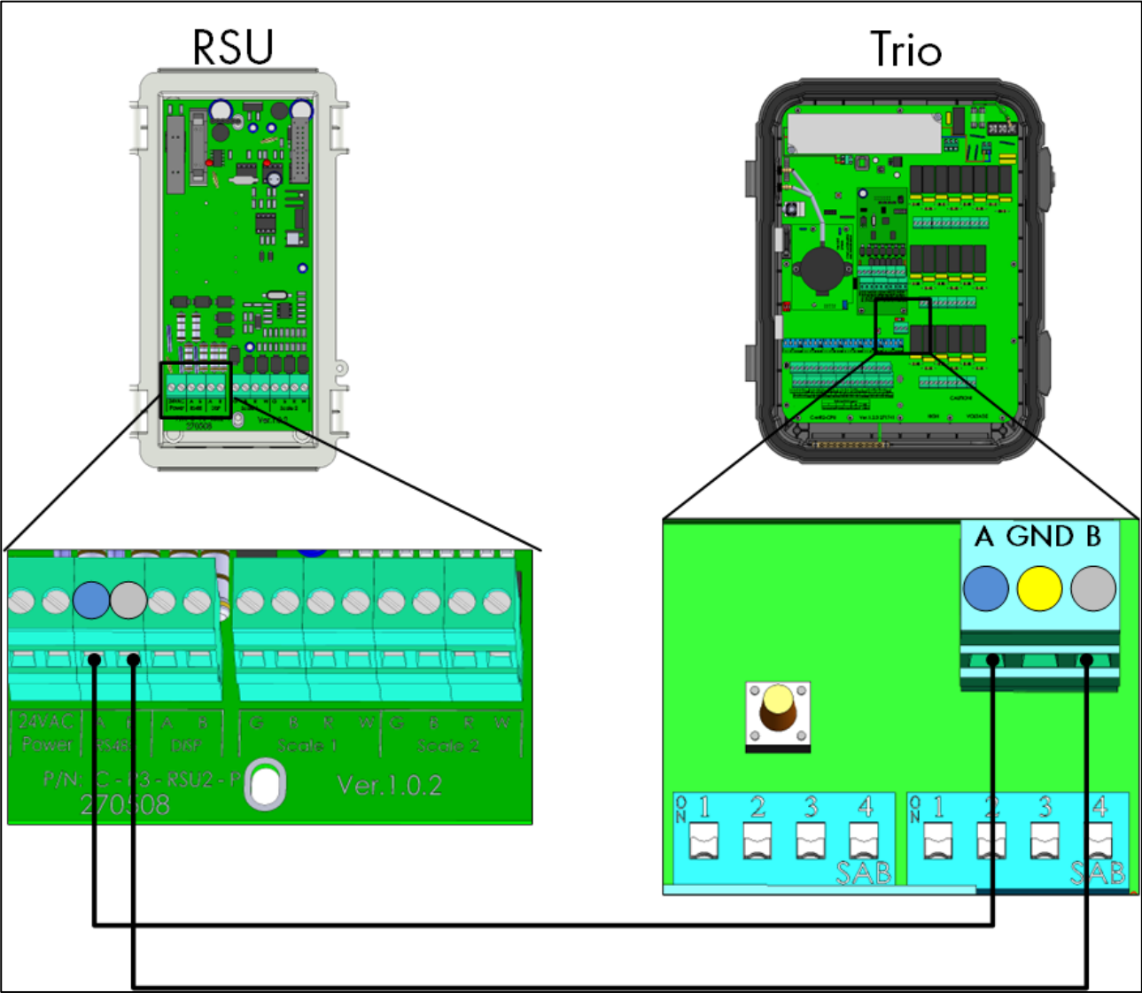
图 43 : Trio和RSU的接线图。
