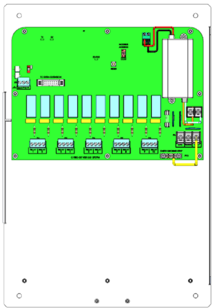
图 62： Trio 扩展继电器面板（正视图）
