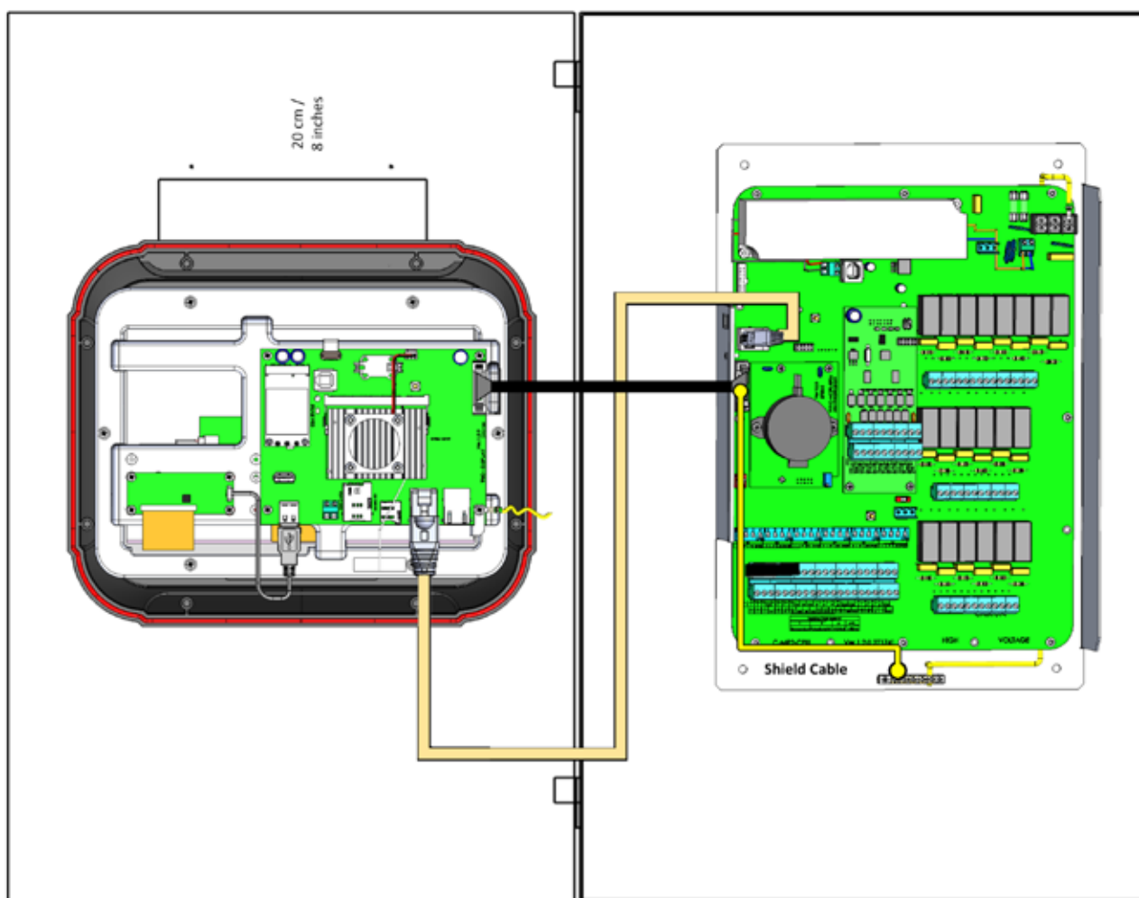
图 59：面板安装， 机柜打开（尺寸不按比例）
