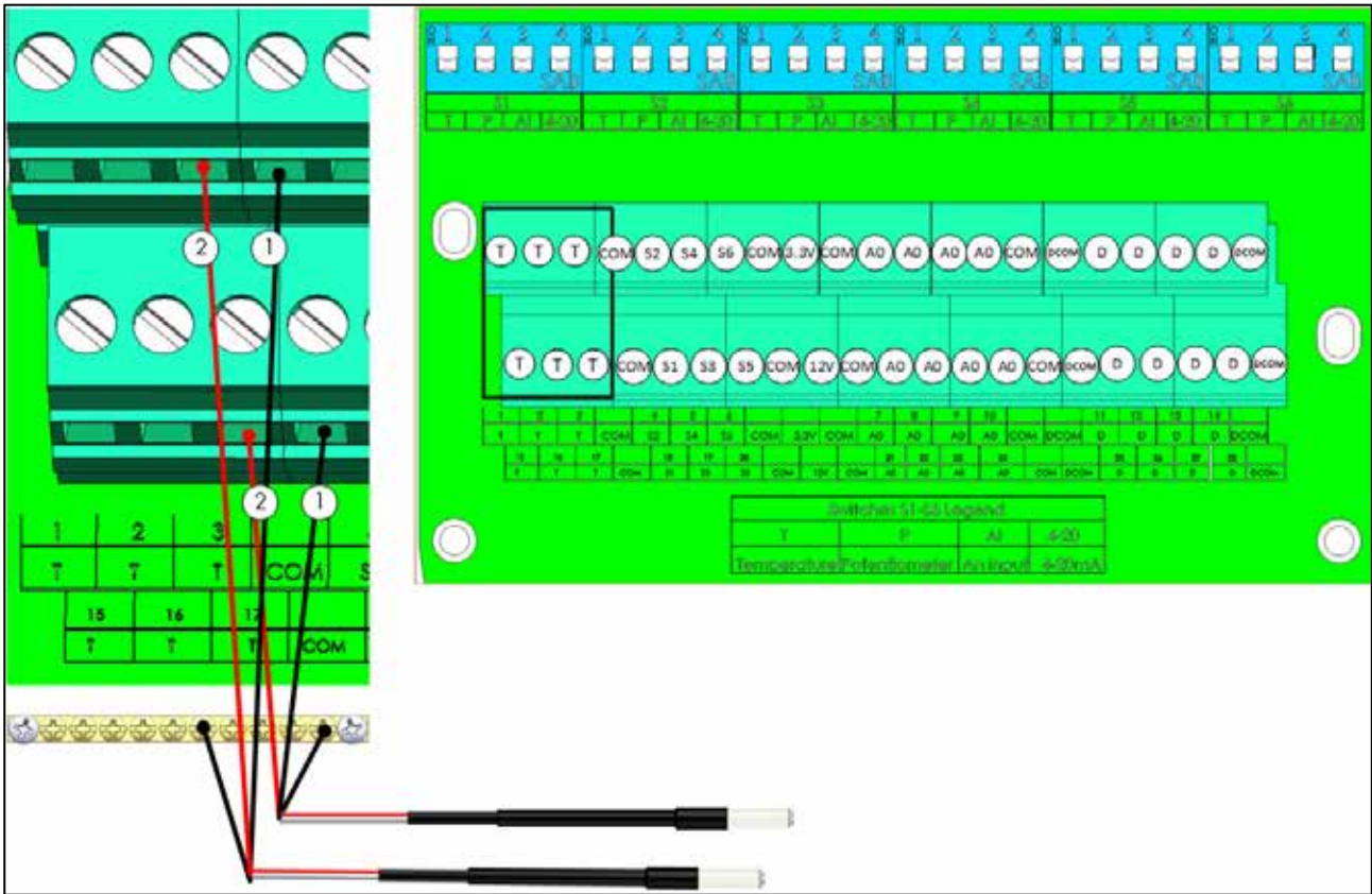
图 23：RTS线
