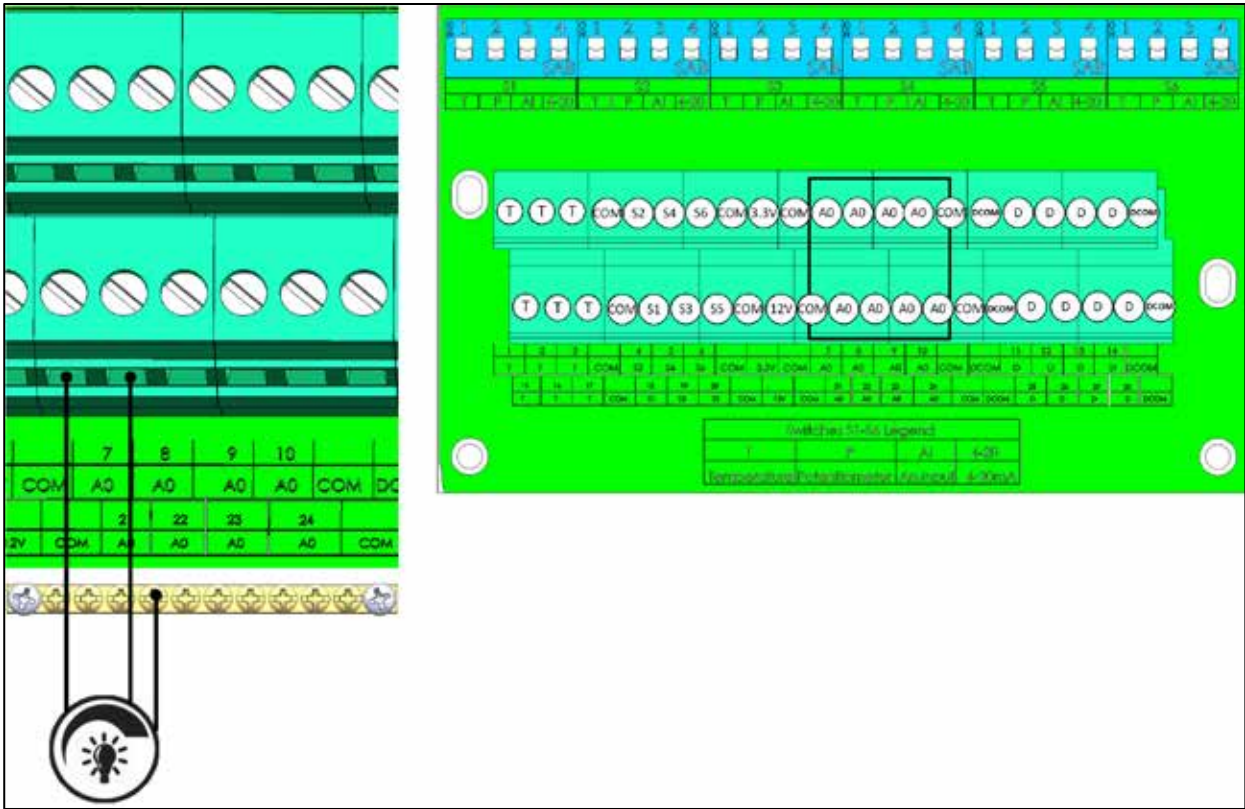
图 17：调光设备
