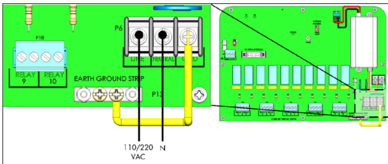
图 66：电源端口
