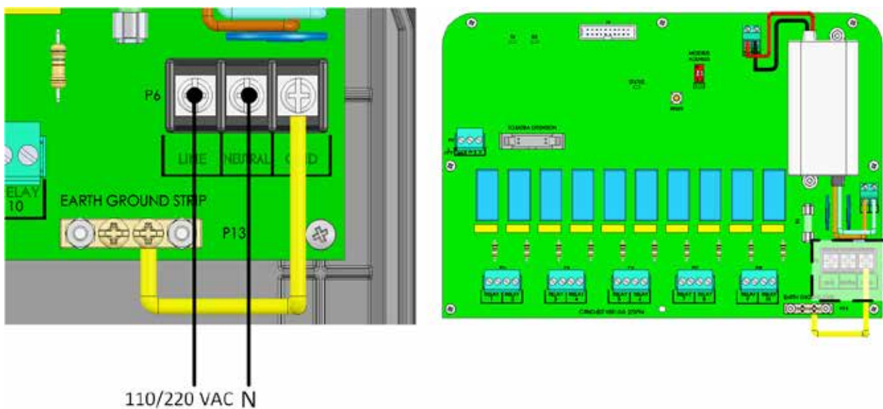
图 52：电源端口
