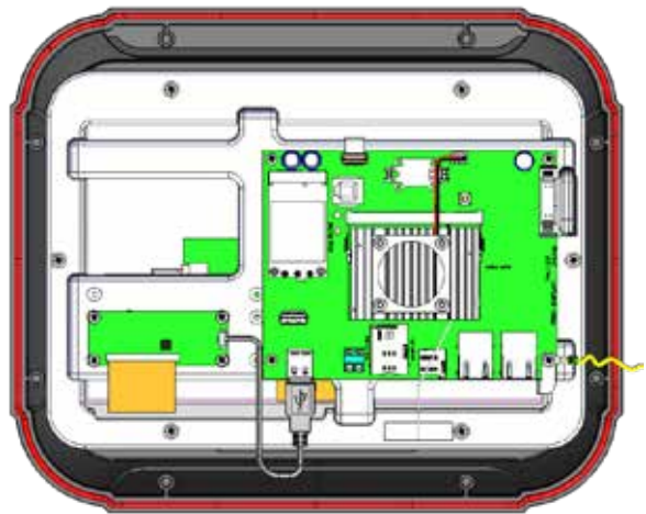
图 54: Trio CPU 面板 (后视图)
