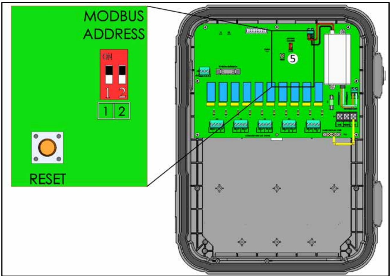
图 49：扩展地址
