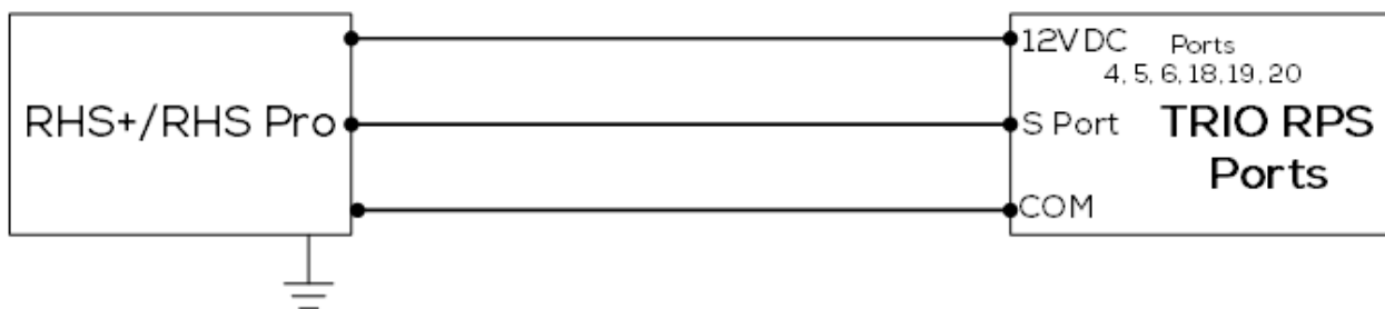
图 29：RHS+/RHS PRO传感器接线图（转换文本）
