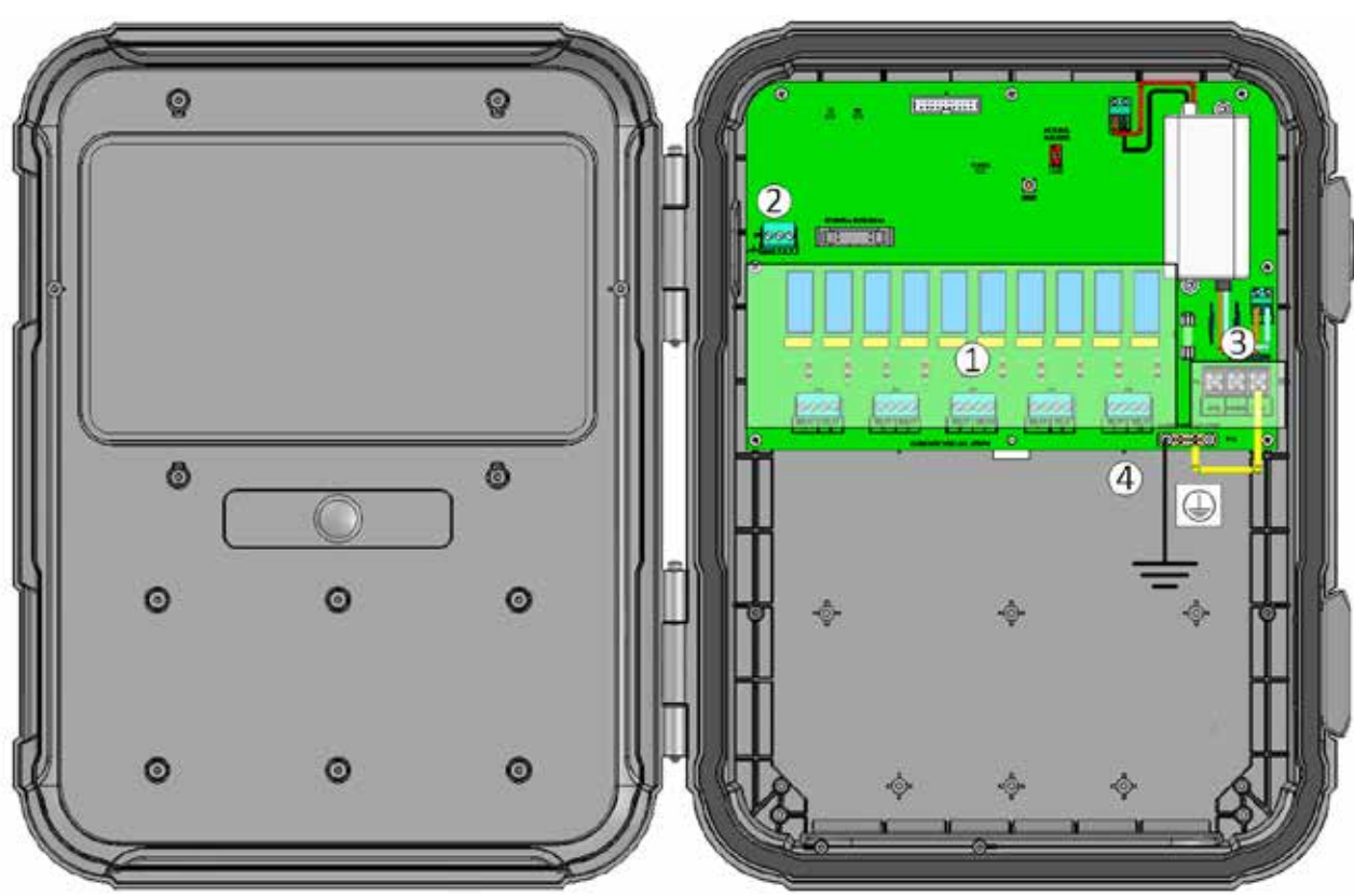
图 47：电路板布局 (转换文本)
