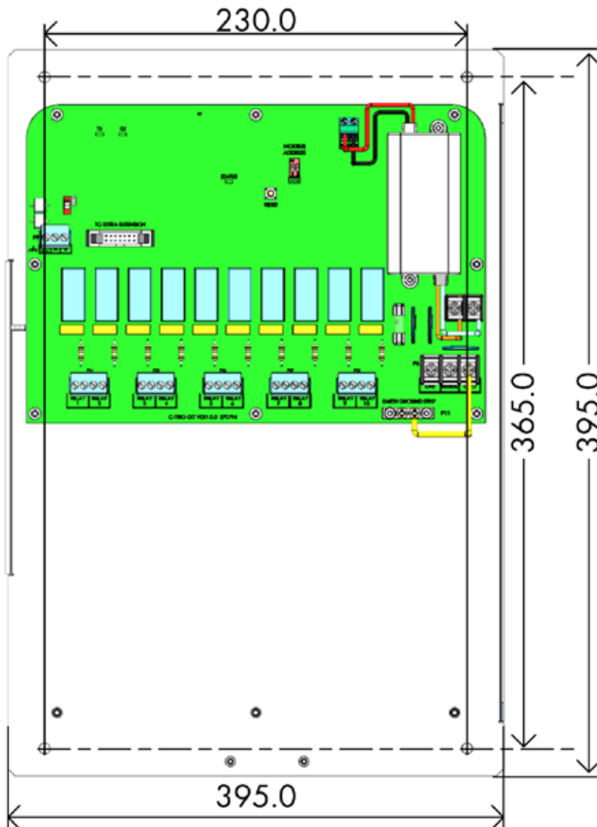
图 63：扩展后面板尺寸
