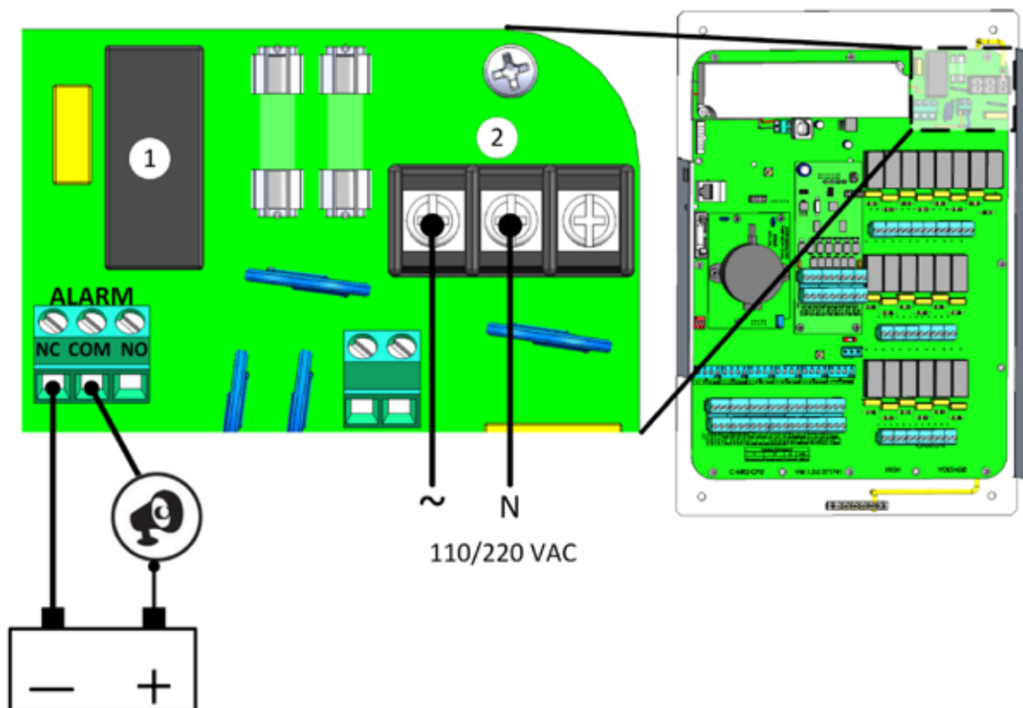
图 60：报警继电器和电源端口
