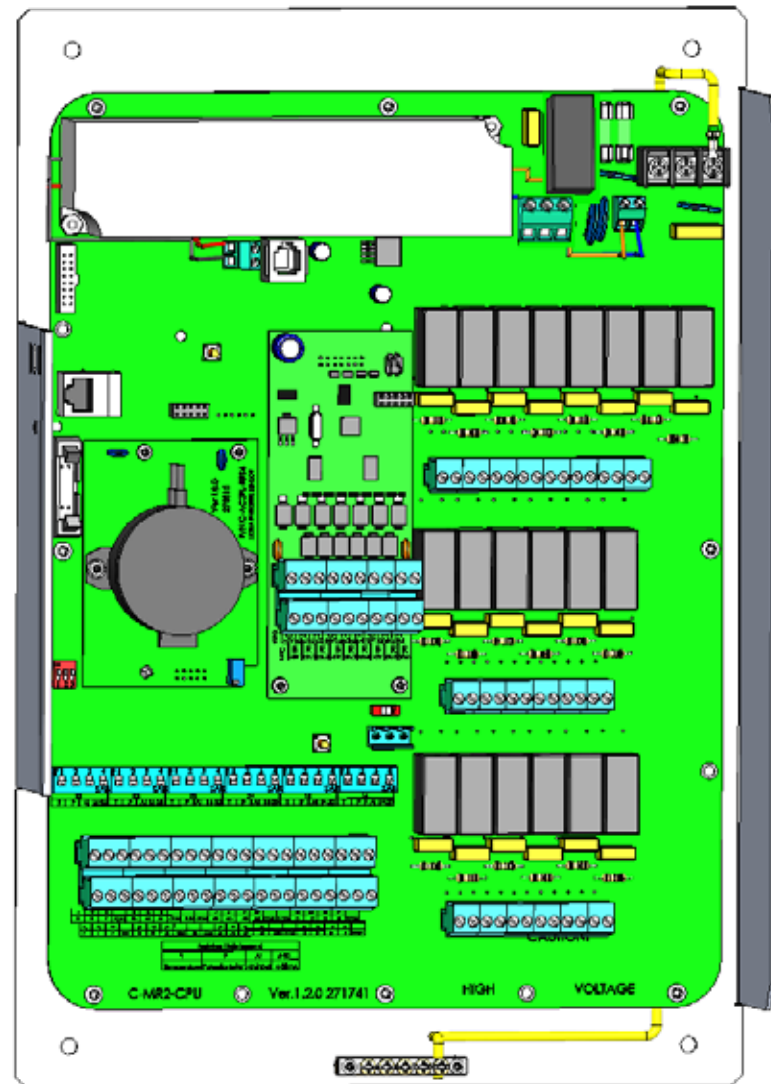
图 55: Trio 继电器面板 e (正视图)
