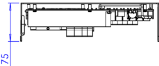
图 57: 后面板深度尺寸
