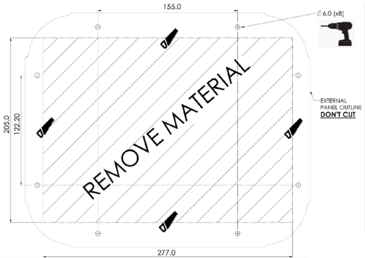
图 58：面板切割和钻孔尺寸（毫米）
