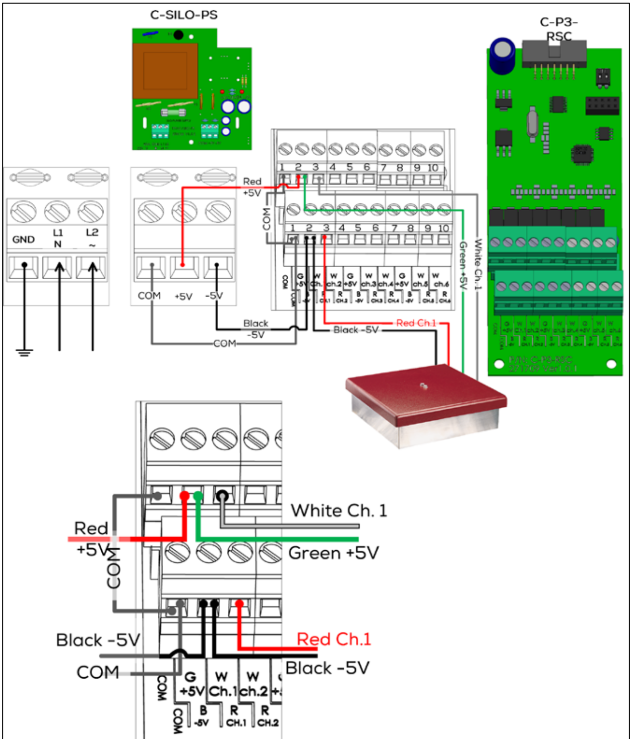
图 39：称重卡接线到电源和鸡秤
