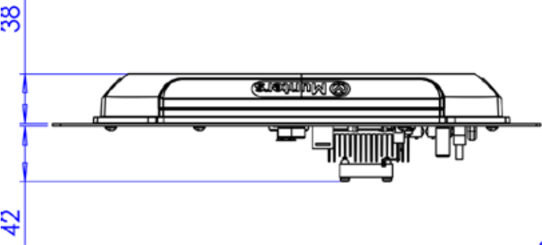
图 2: 前面板深度尺寸
