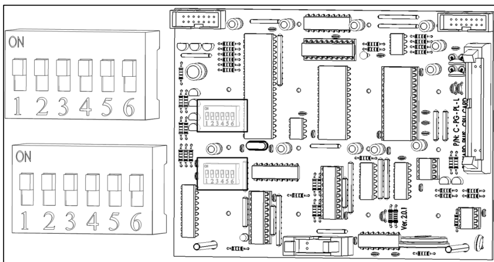
图 13: Pig Guard Plus的 CPU
