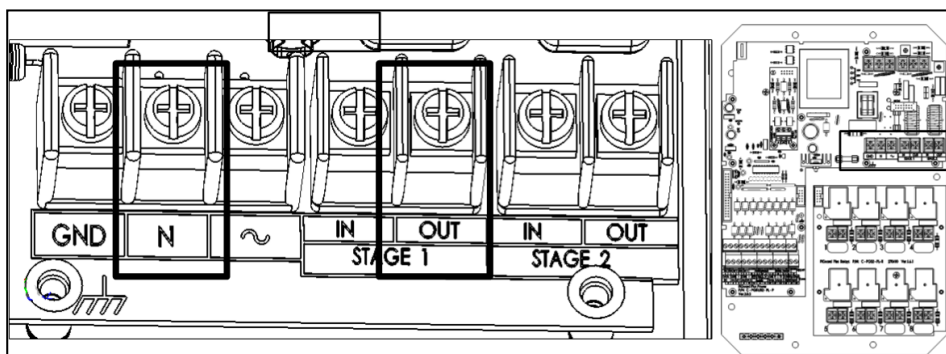
图 4: 可控硅1电源
