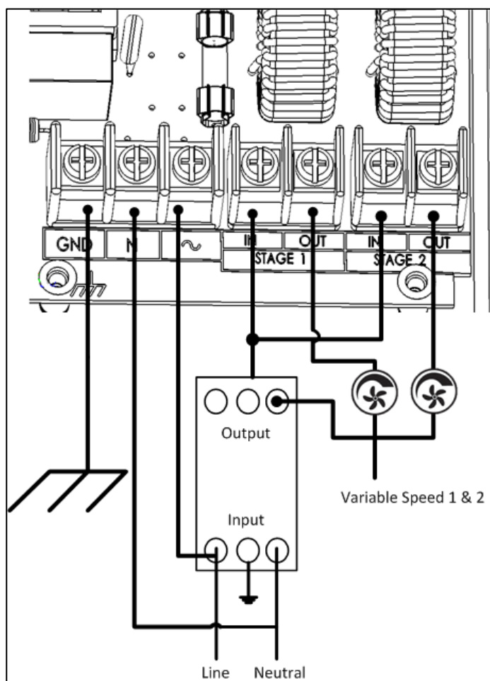
图 11: 电源接线示意图
