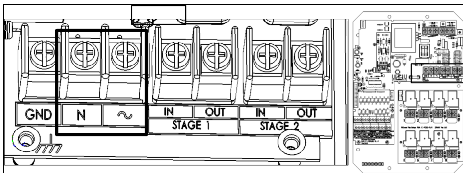
图 3: 电源输入端
