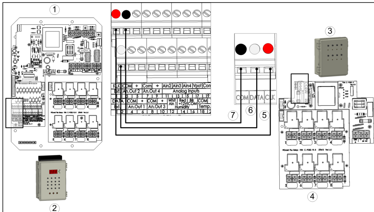
图 14: Pig Guard Plus扩展盒接线示意图
