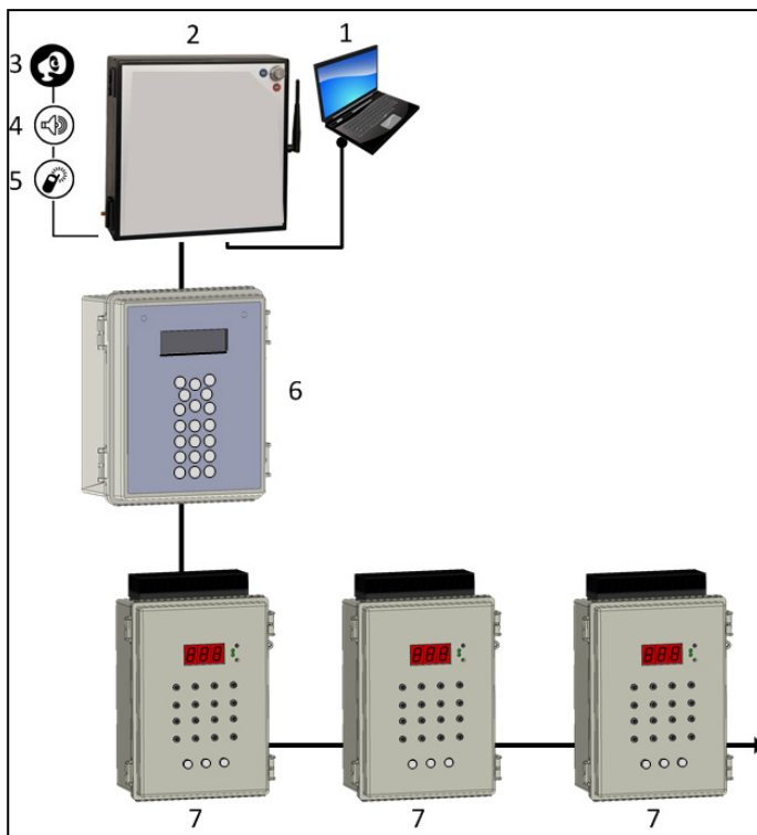
图 2: Super Guard - Pig Guard Plus - 通信器联网示意图
