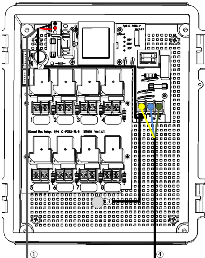
图 15: 扩展盒布线
