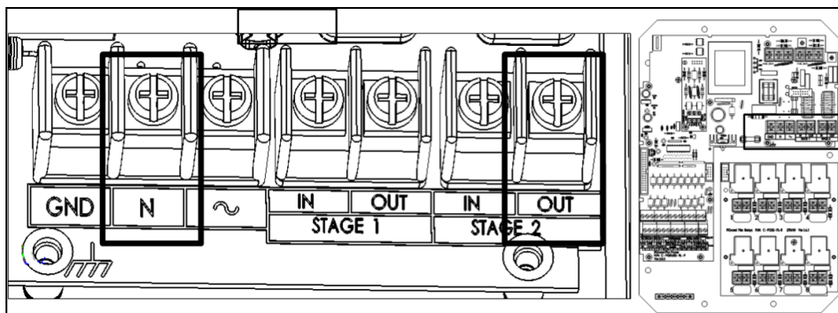
图 5: 可控硅2电源
